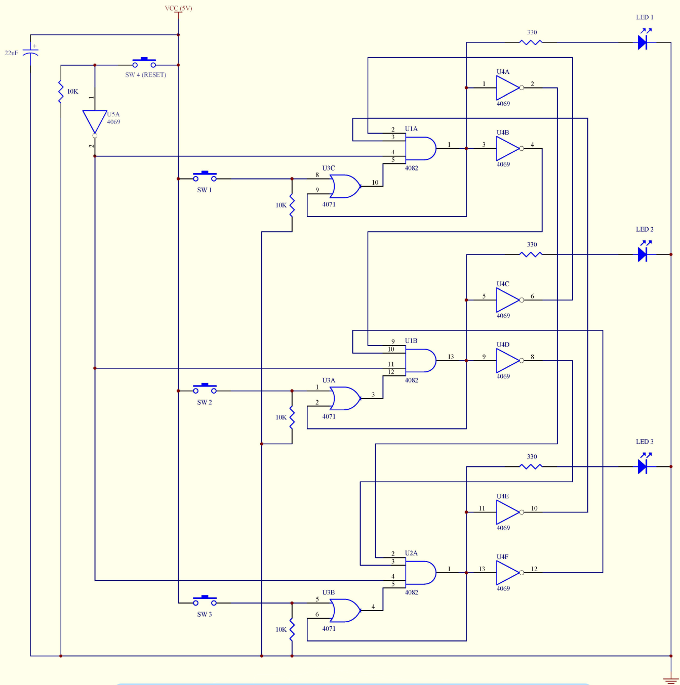
三人搶答系統 (進階版) 參考電路 Advanced Quick Answering System (3 Participants)
