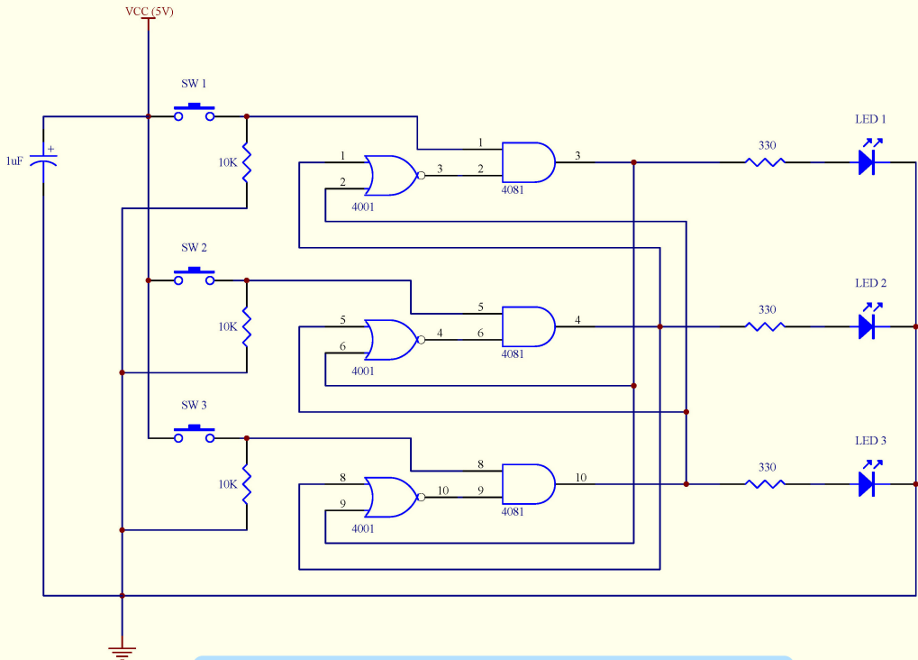
三人搶答系統 (初階版) 參考電路 Simplified Quick Answering System (3 Participants)
